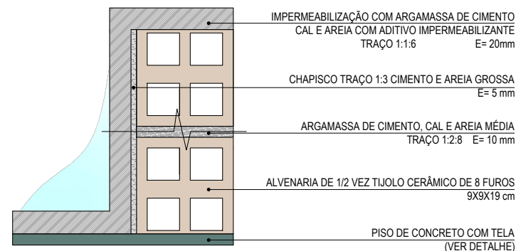
Detalhe – Impermeabilização escala 1/5
