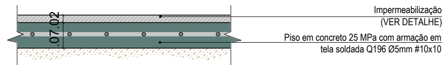
Detalhe – Piso de conc. com tela escala 1/10
