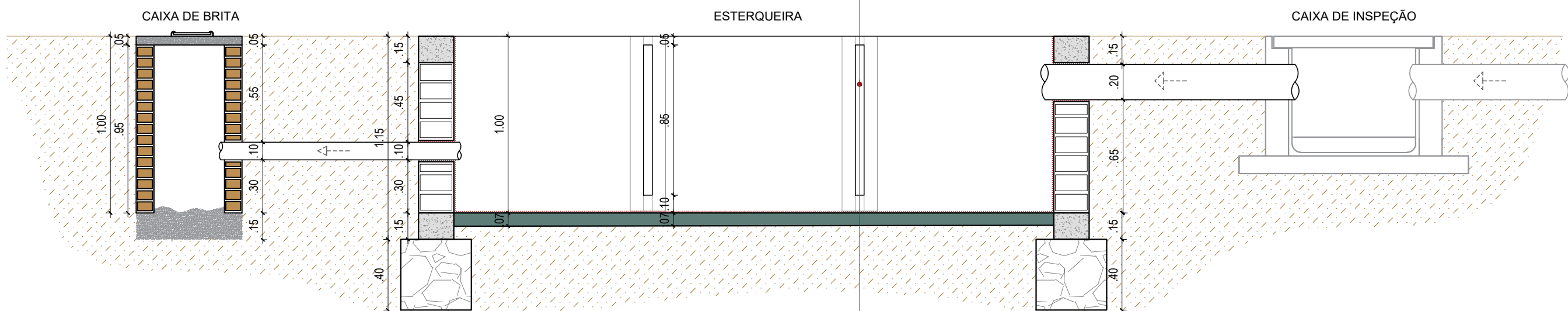
Corte Longitudinal – AA escala 1/25
