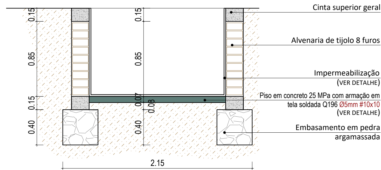
Corte BB – Transversal escala 1/25
